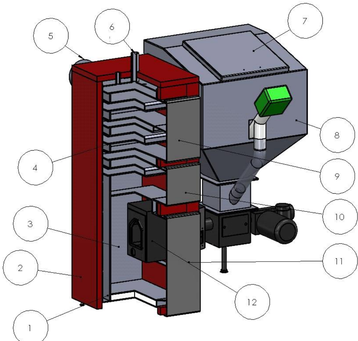
Rys.1. Kocioł "Technix-Pel"
